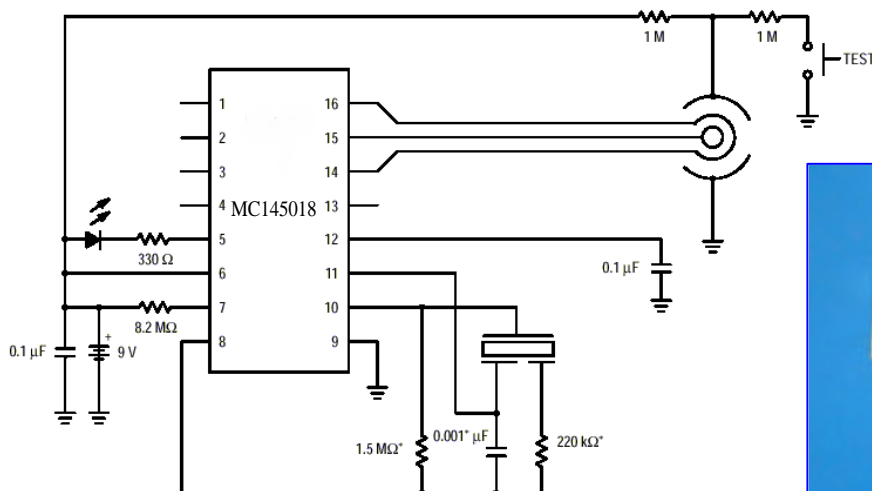
采用 MC145018 的烟雾探测器电原理图
