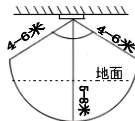
(吸顶安装图示)
